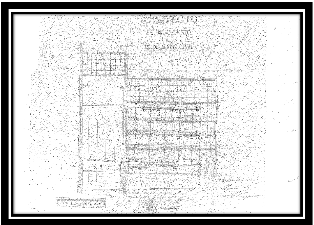
Ilustración 21: Sección longitudinal
