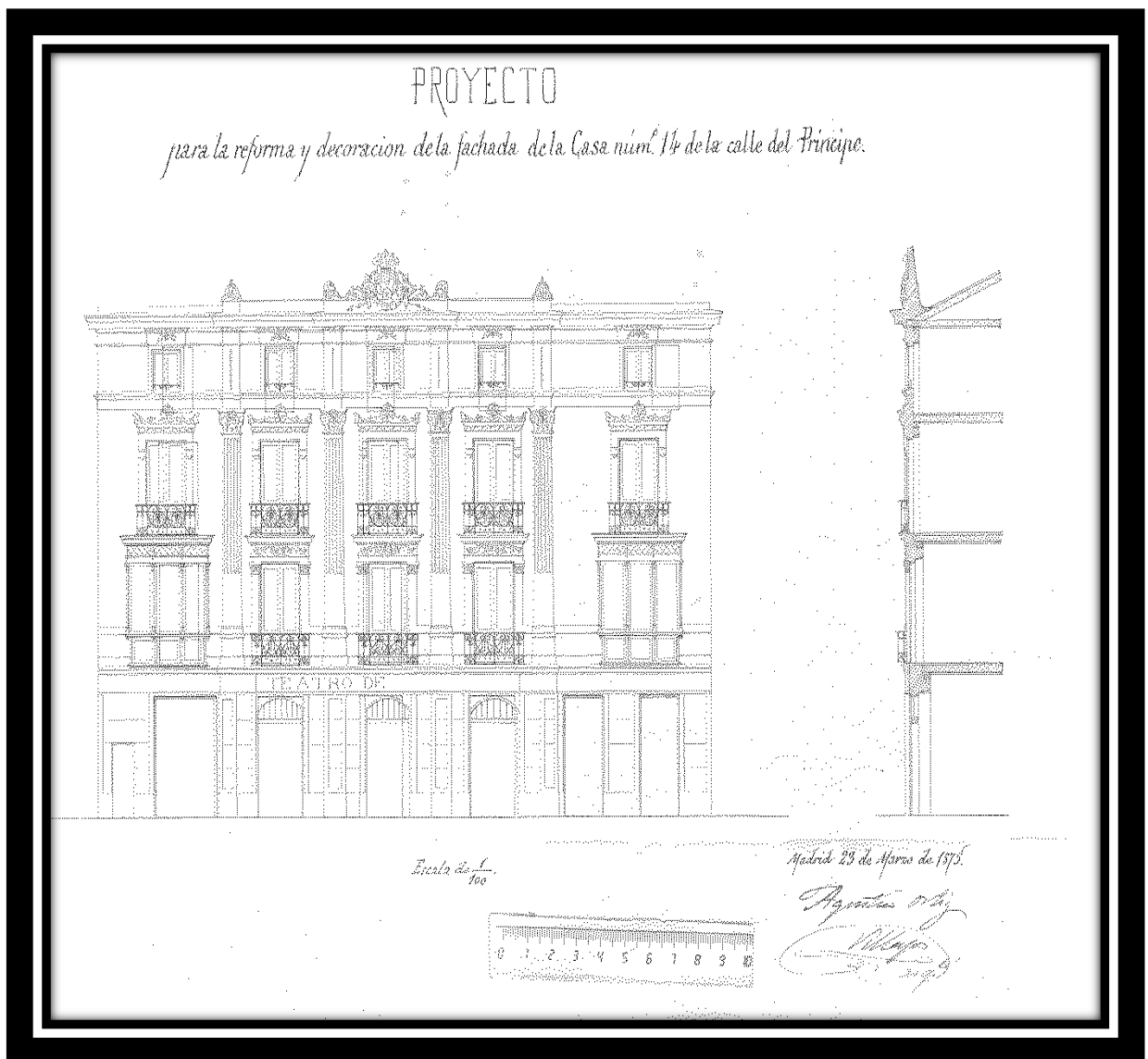
Ilustración 22: Fachada
