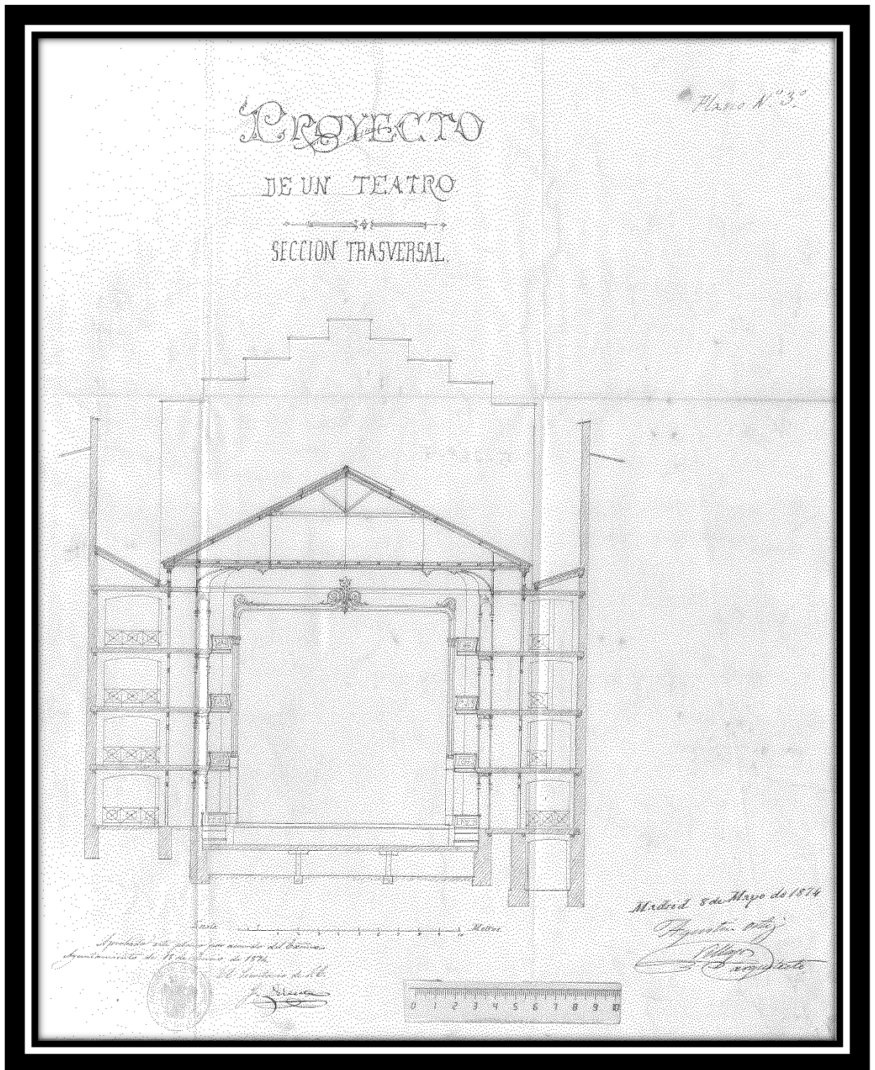
Ilustración 23: Sección trasversal
