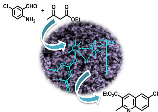
Figura 3. Esquema gráfico de la reacción Friedländer catalizada por nanopartículas de \text{Co}^0 soportadas en aerogeles de carbón.
