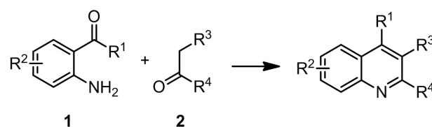
Esquema 1. Condensación de Friedländer entre 2-aminoarilaldehídos/cetonas (1) y compuestos carbonílicos con grupos metilenos activos (2).
