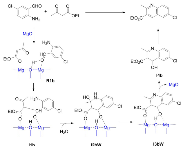
Esquema 2. Mecanismo de reacción propuesto para la condensación entre 2-amino-5-clorobenzaldehído y acetilacetato de etilo catalizada por un clúster de MgO.
