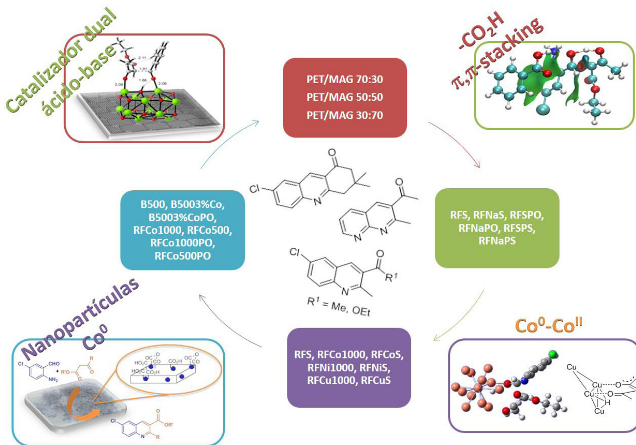
Figura 4. Resumen gráfico de los cuatro capítulos de esta Tesis Doctoral.
