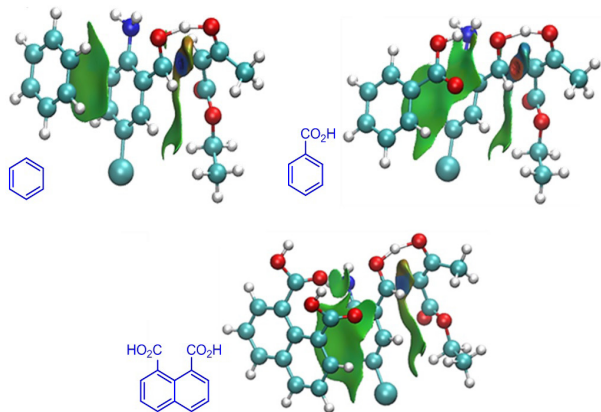
Figura 2. Representación de las interacciones \pi,\pi -stacking mediante el gráfico NCI en la etapa de formación del enlace C-C para cada uno de los modelos catalíticos estudiados.
