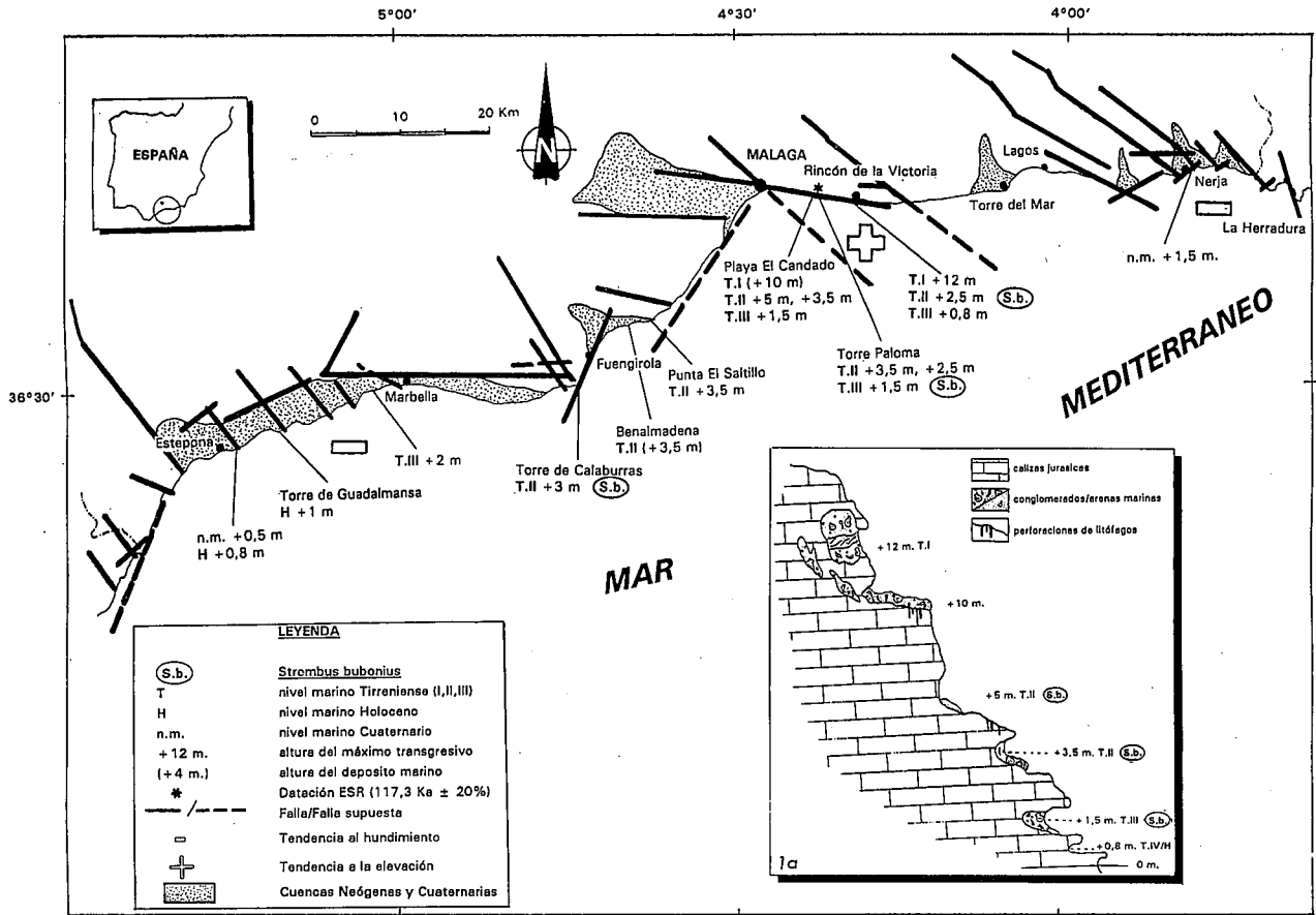
Figura 1.- Distribución de los episodios marinos cuaternarios de la costa de Málaga (Episodios Tirrenienses y Holoceno). con indicación de las fallas más importantes que controlan las alturas de los máximos transgresivos. 1a. Secuencia tipo de los episodios marinos del Pleistoceno medio-superior y Holoceno en el sector Málaga-Rincón de la Victoria.
