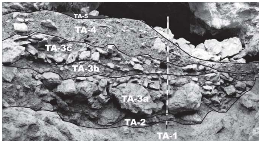
Fig. 2.- Stratigraphical scheme of Torca l'Arroyo.
